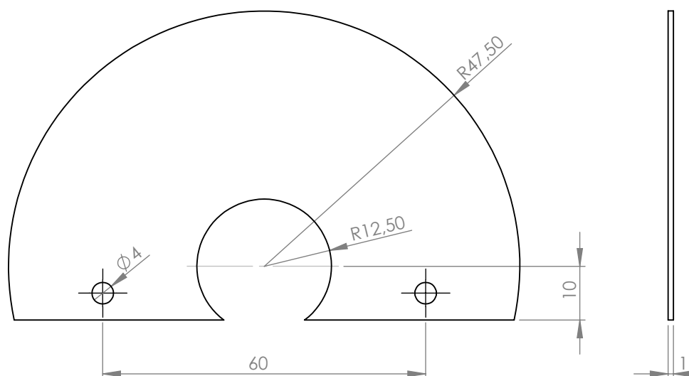
Apoio frontal Escala 1:1
